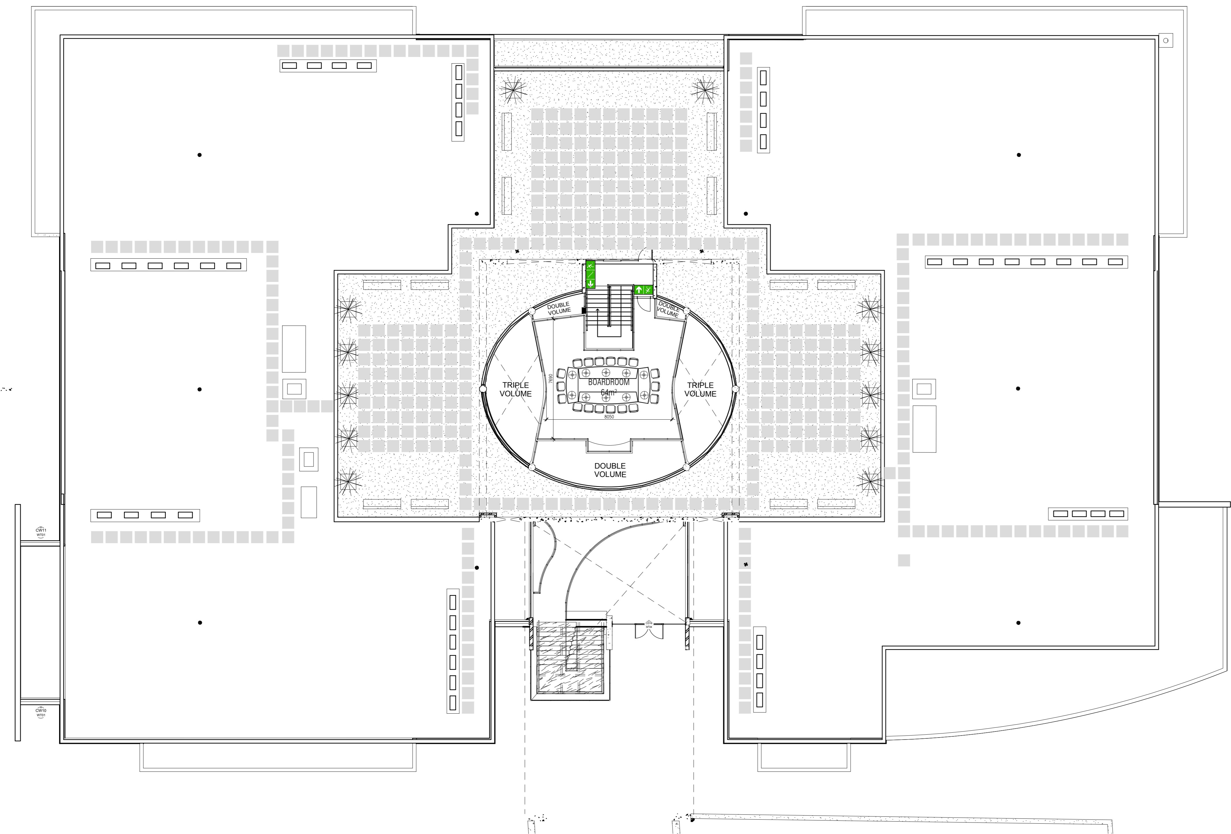
1 TENANT INSTALLATION 223 1:200 MEZZANINE FLOOR
